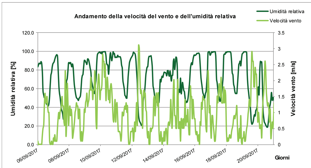
Fig. 2.1/F – Andamento dei parametri velocità del vento e umidità relativa, rilevati presso la stazione di monitoraggio ATM-LE-01 (periodo 06/09/2017 – 21/09/2017)
