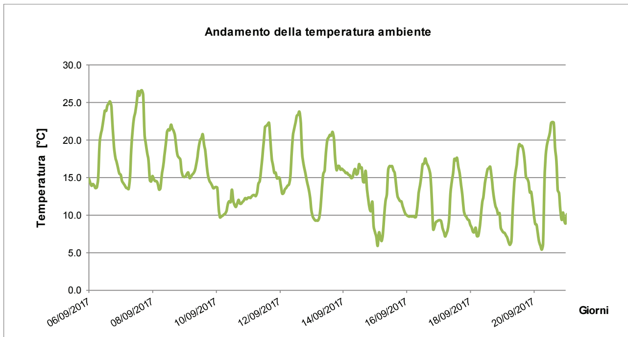
Fig. 2.1/E – Andamento della temperatura rilevata presso la stazione di monitoraggio ATM-LE-01 (periodo 06/09/2017 – 21/09/2017)
