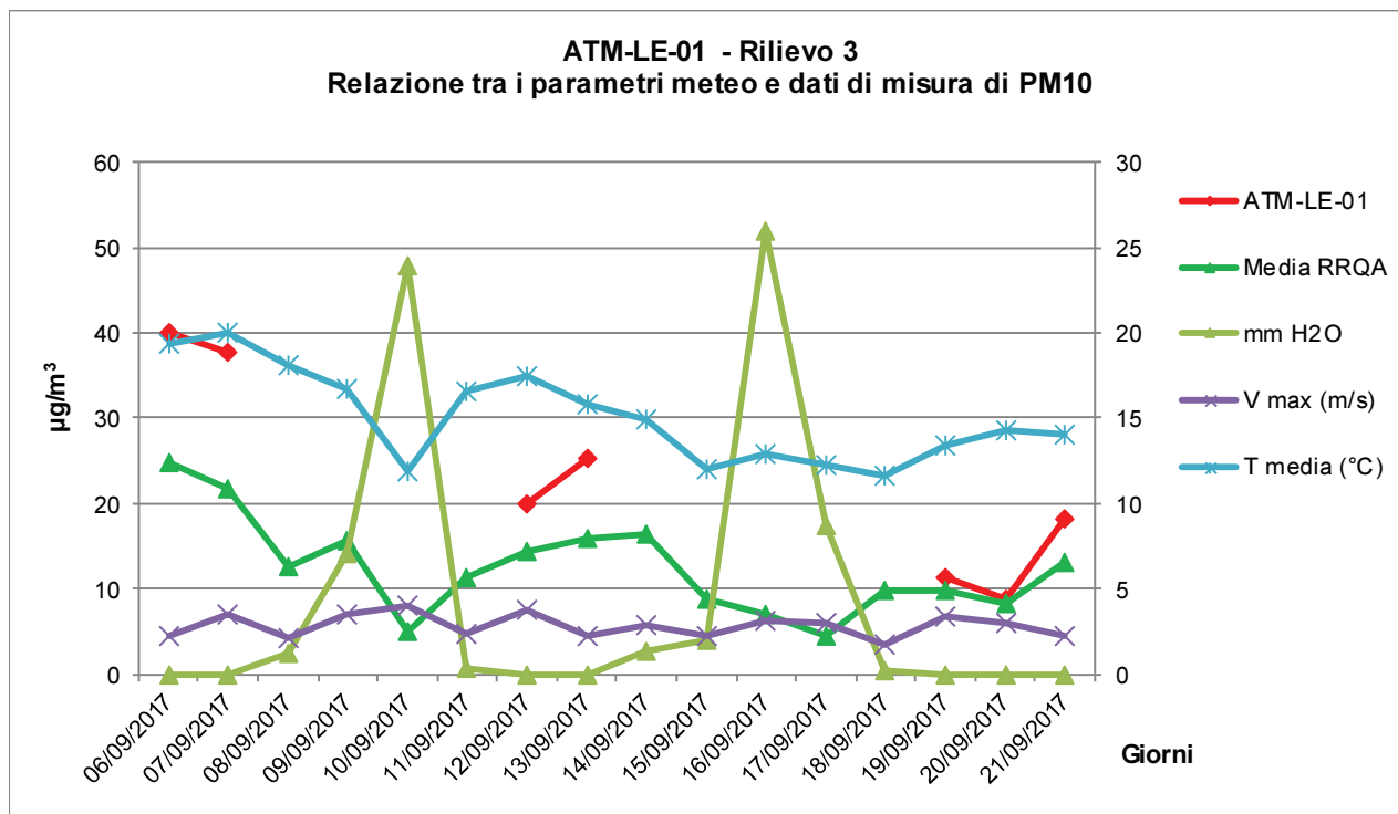
Fig. 2.2/F – Andamento delle concentrazioni di PM10 e dei parametri meteo presso la postazione ATM-LE-01 e presso le centraline ARPA dal 06/09/2017 al 21/09/2017
