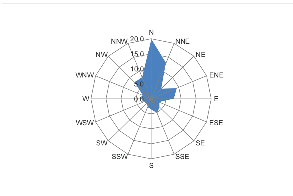
Fig. 2.1/G – Andamento della rosa dei venti, costruita sulla base dei dati rilevati presso la stazione di monitoraggio ATM-LE-01 (periodo 06/09/2017 – 21/09/2017)
