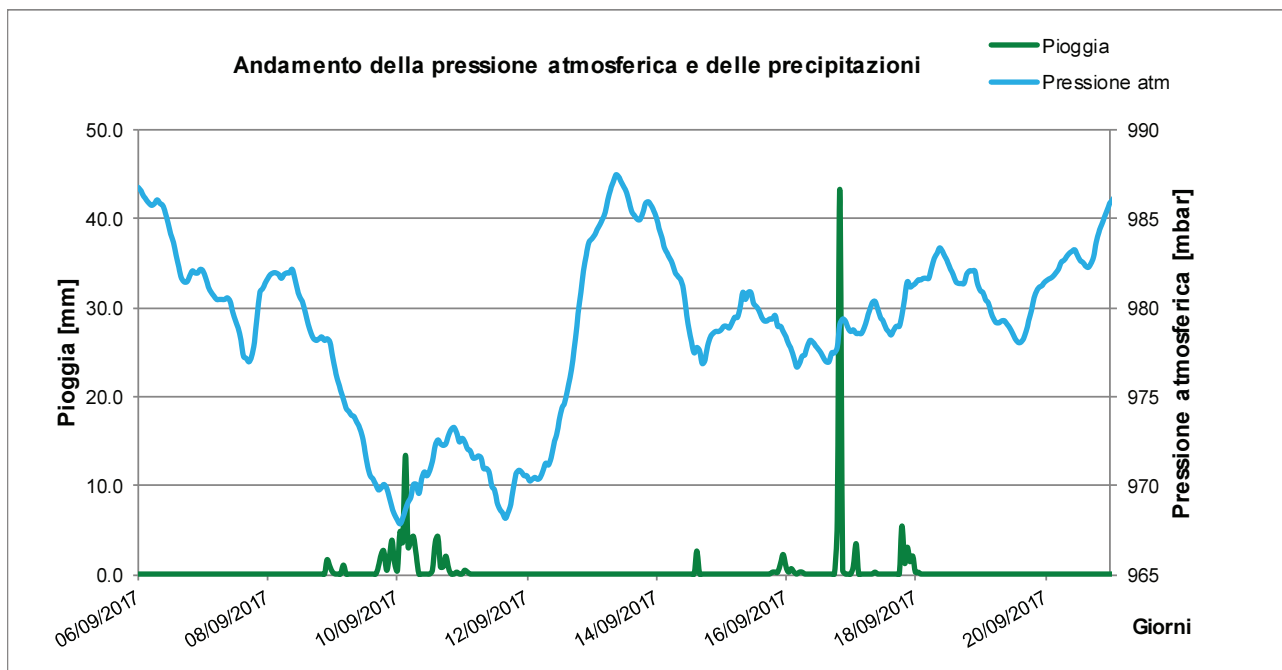
Fig. 2.1/D – Andamento dei parametri pressione atmosferica e precipitazioni, rilevati presso la stazione di monitoraggio ATM-LE-01 (periodo 06/09/2017 – 21/09/2017)
