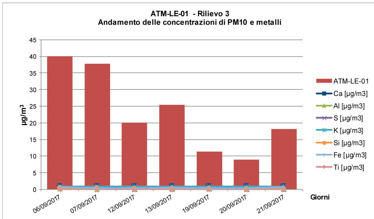
Fig. 2.2/B – Andamento delle concentrazioni di PM10 e di metalli terrigeni rilevate presso la postazione ATM-LE-01 dal 06/09/2017 al 21/09/2017
