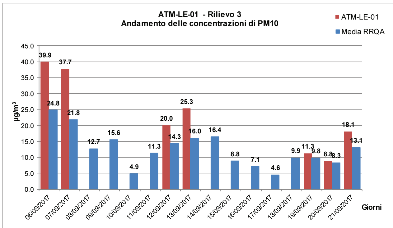
Fig. 2.2/E – Andamento delle concentrazioni di PM10 presso la postazione ATM-LE-01 e presso le centraline ARPA dal 06/09/2017 al 21/09/2017
