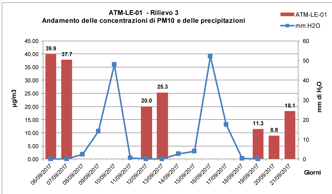
Fig. 2.2/A – Andamento delle concentrazioni di PM10 e delle precipitazioni rilevate presso la postazione ATM-LE-01 dal 06/09/2017 al 21/09/2017
